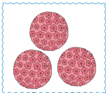
Vi-rút HPV
